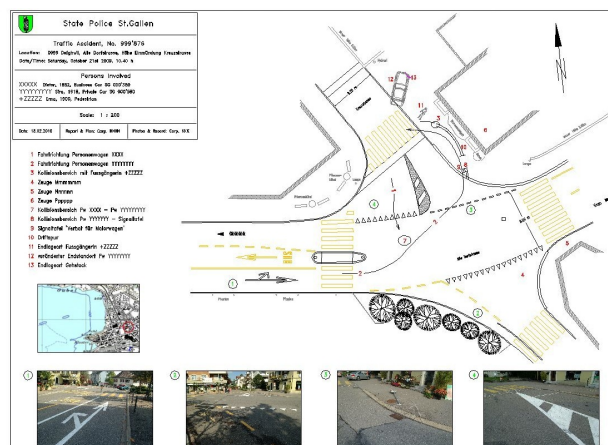
Maßstäbliche Zeichnung eines Verkehrsunfalls: Endlage der Fahrzeuge und Bremsspuren.
